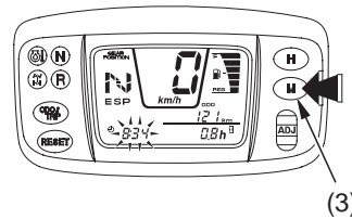
(3) minuuttien valintapainike
